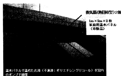
図2 ログハウス型木材乾燥室(兵庫県森林技術センター)
