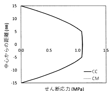
図 9 スギ CLT およびセンダン複合 CLT の破壊時の応力分布：上：曲げ応力、下：せん断応力
